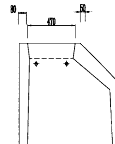
側面図
