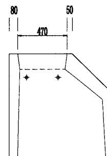
右側面図
