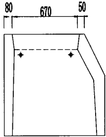
左側面図
