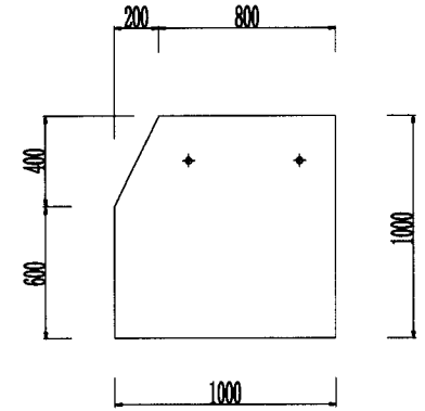
右側面図
