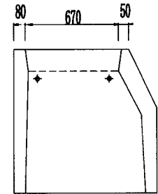
右側面図
