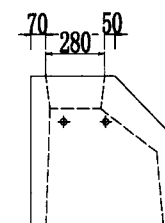
端面図
