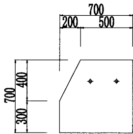
端面図
