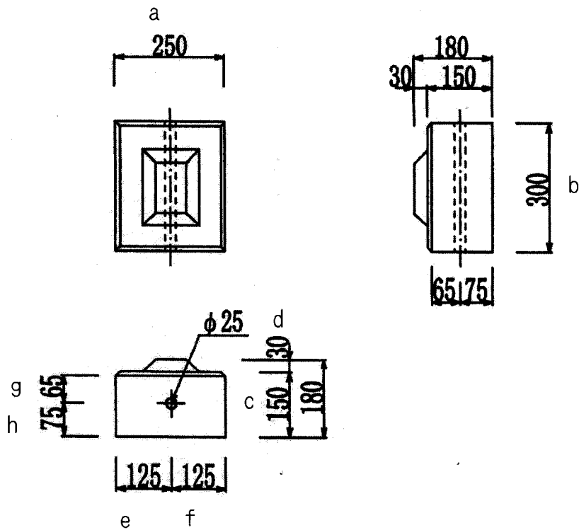
連節ブロック 半長型 250×300×150
