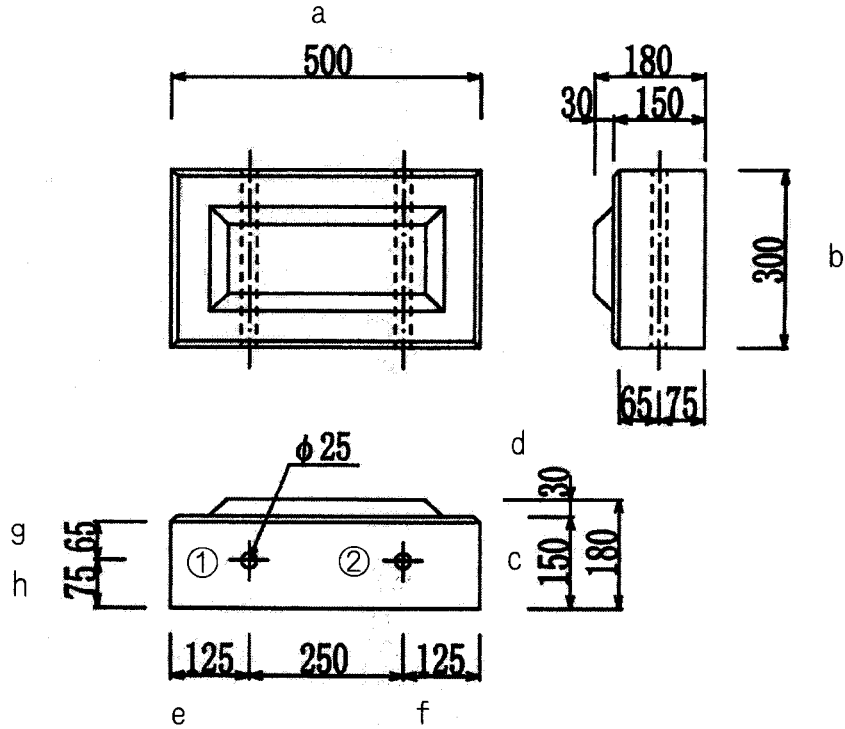
連節ブロック 基本型 500×300×150
