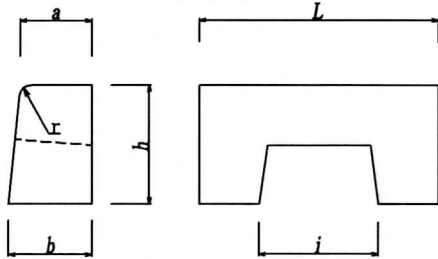
片面歩車道境界ブロック (水抜き)
