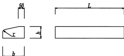
身障者境界ブロック
