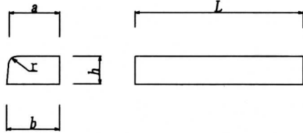
片面歩車道境界ブロック (乗り入れ)
