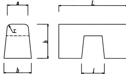
両面歩車道境界ブロック (水抜き)
