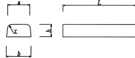
両面歩車道境界ブロック (乗り入れ)
