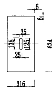
側面図
